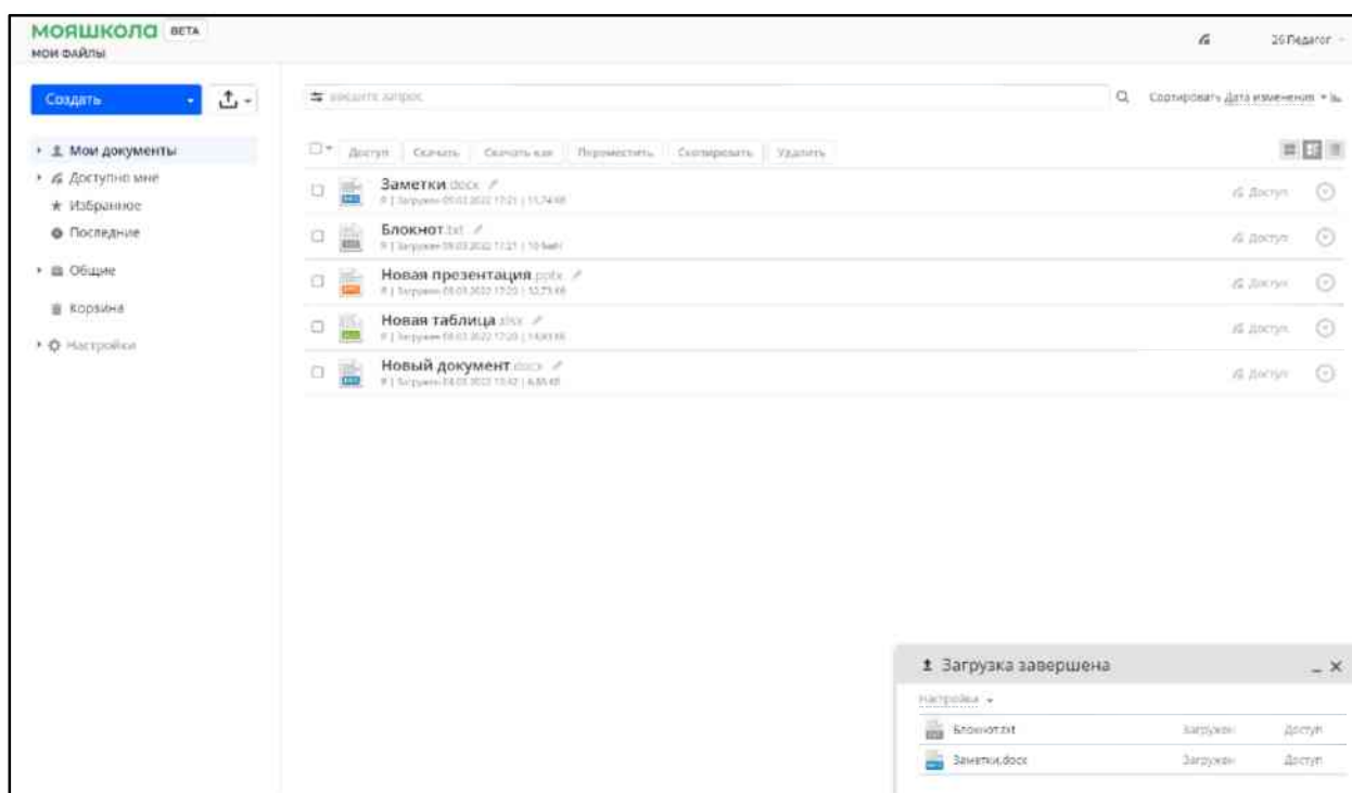
Рисунок 13 – Загрузка файла
